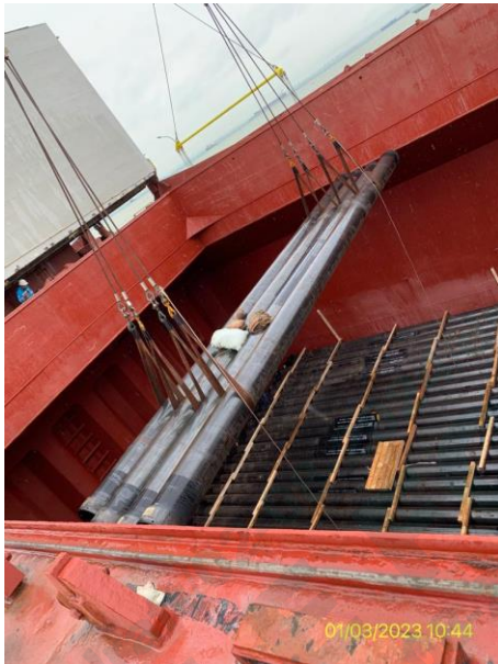
Hold № 2 Cargo Loading
