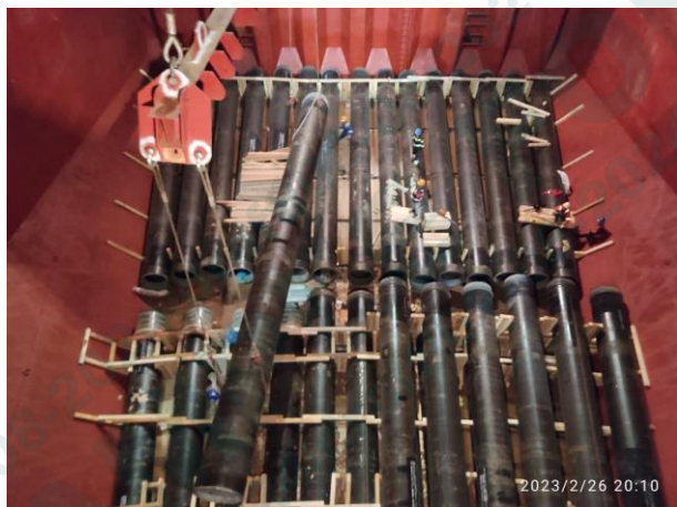
Hold № 4 Cargo Loading
